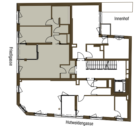
Geschossplan
