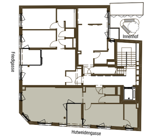
Geschossplan
